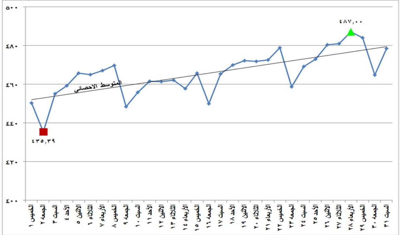
شكل (١٥) إجمالي الطاقة الكهربائية المنتجة من كل المصادر الأولية خلال شهر ديسمبر ٢٠١٦
