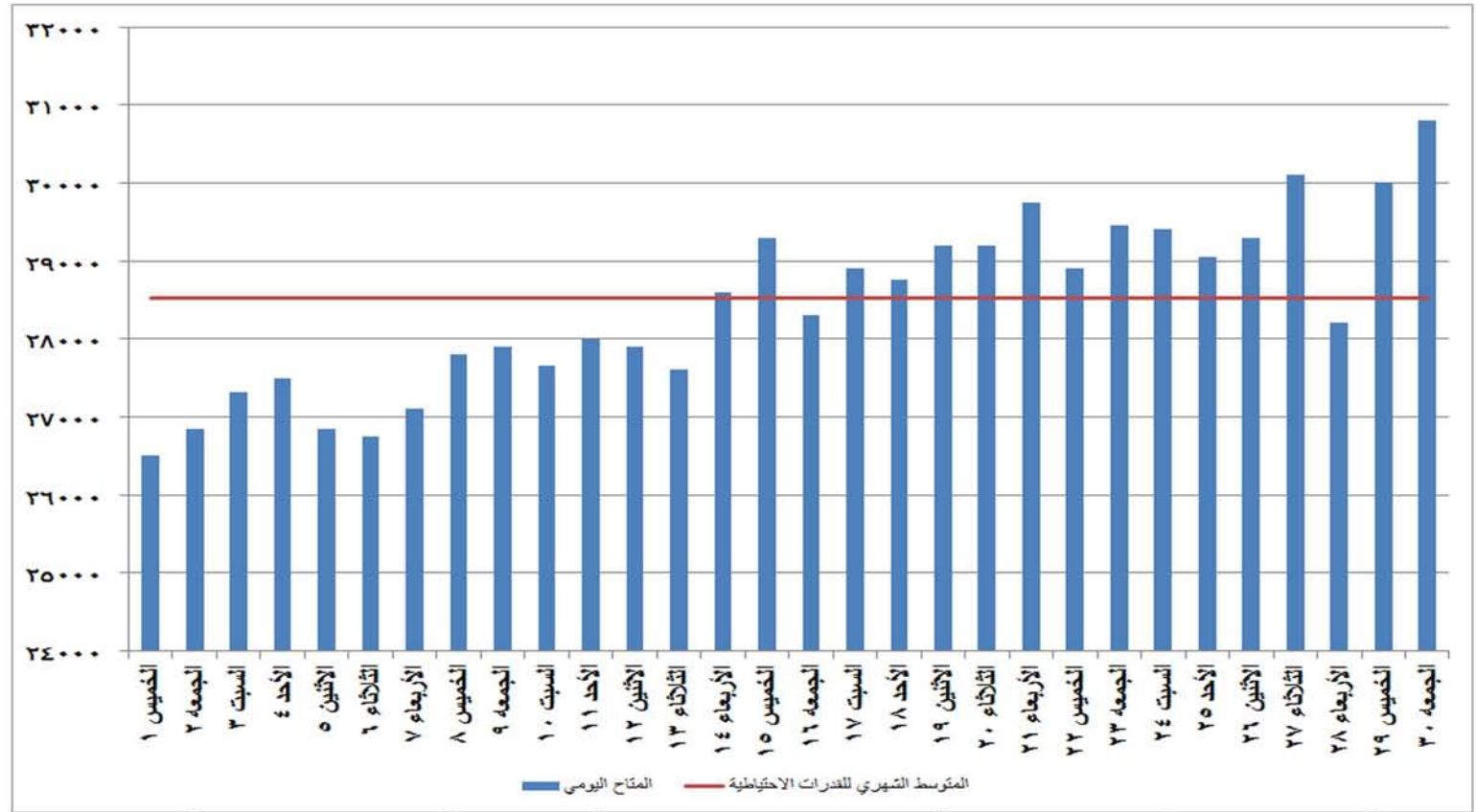
شكل (٢٧) القدرات المتاحة يوميا والمتوسط الشهري للقدرة الاحتياطية خلال شهر ديسمبر ٢٠١٦
