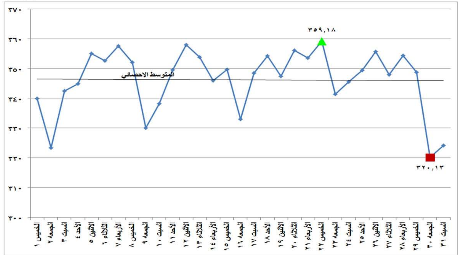
شكل (١٧) الطاقة الكهربائية المنتجة من الغاز الطبيعي خلال شهر ديسمبر ٢٠١٦
