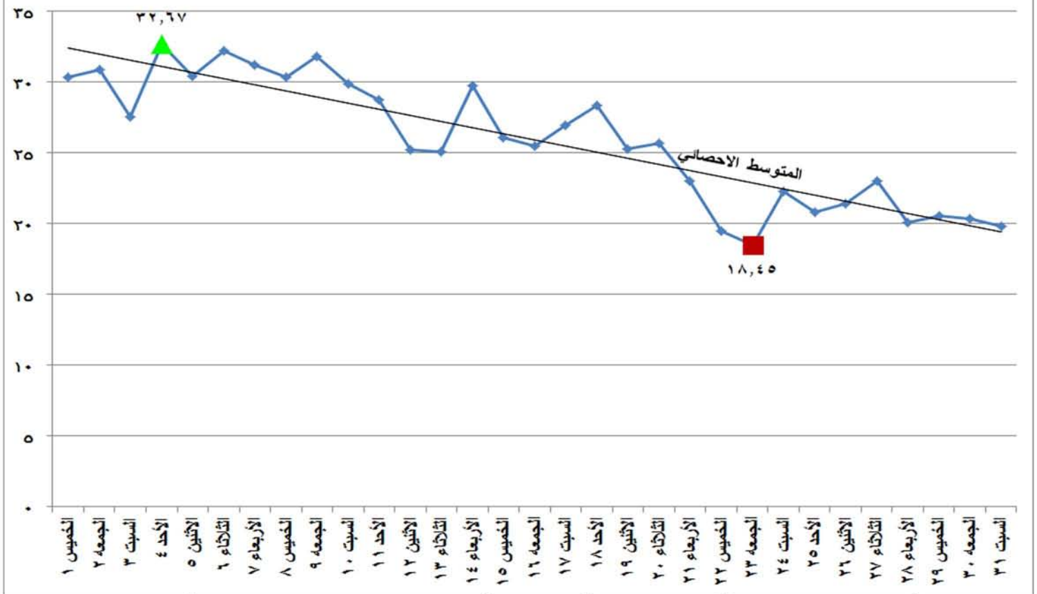
شكل (٢١) الطاقة الكهربائية المنتجة من المصادر غير الحرارية خلال شهر ديسمبر ٢٠١٦
