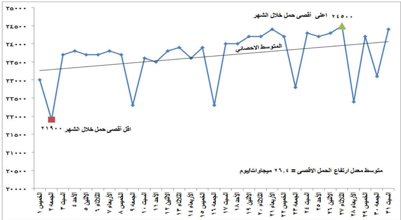
شكل (١) تطور الحمل الاقصى اليومي خلال شهر ديسمبر ٢٠١٦
