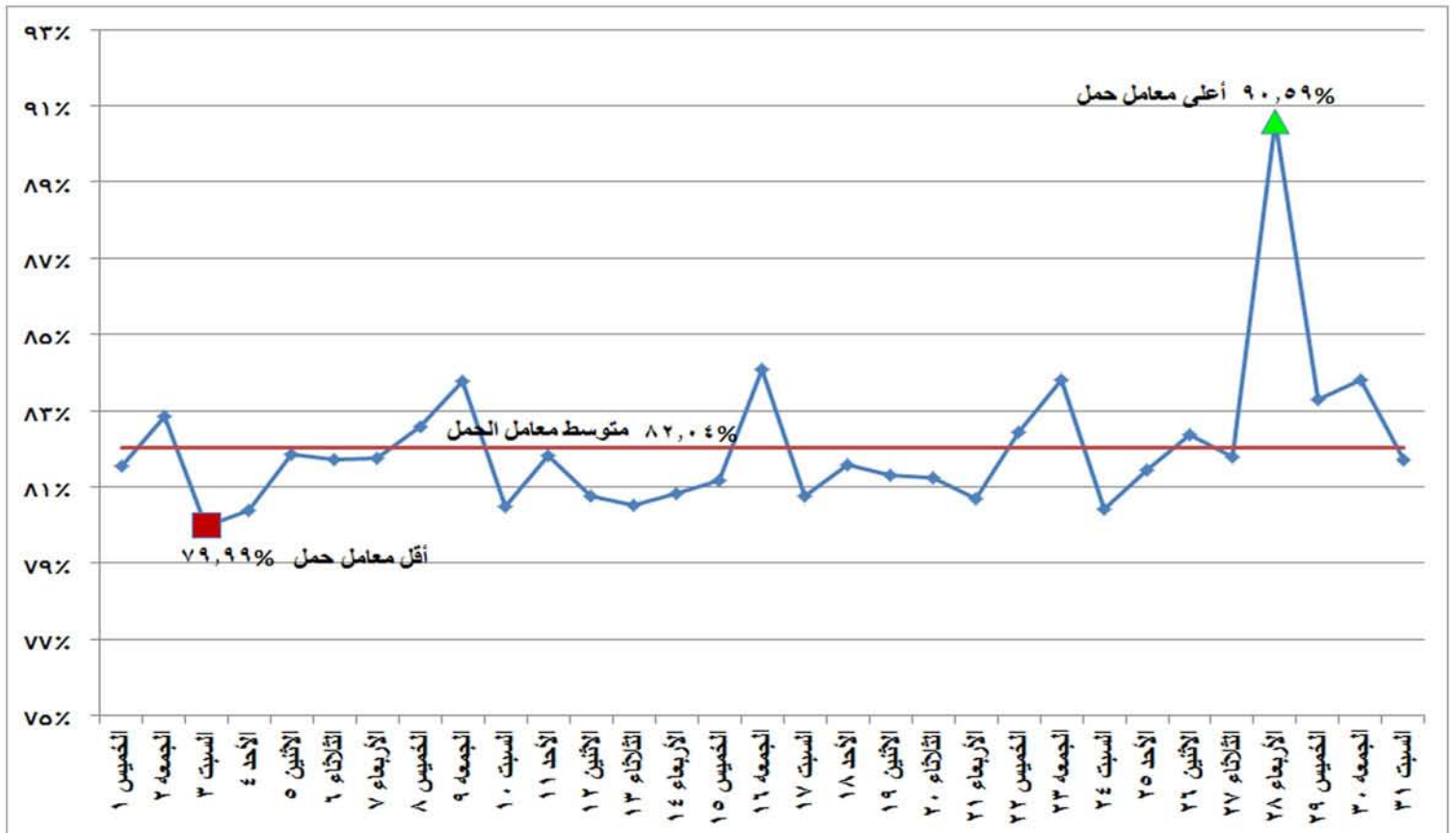
شكل (١٢) إجمالي معامل الحمل لوحدات الانتاج خلال شهر ديسمبر ٢٠١٦
