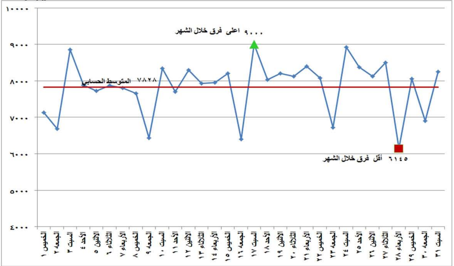
شكل (٣) الفرق بين أقصى وأدنى حمل خلال شهر ديسمبر ٢٠١٦
