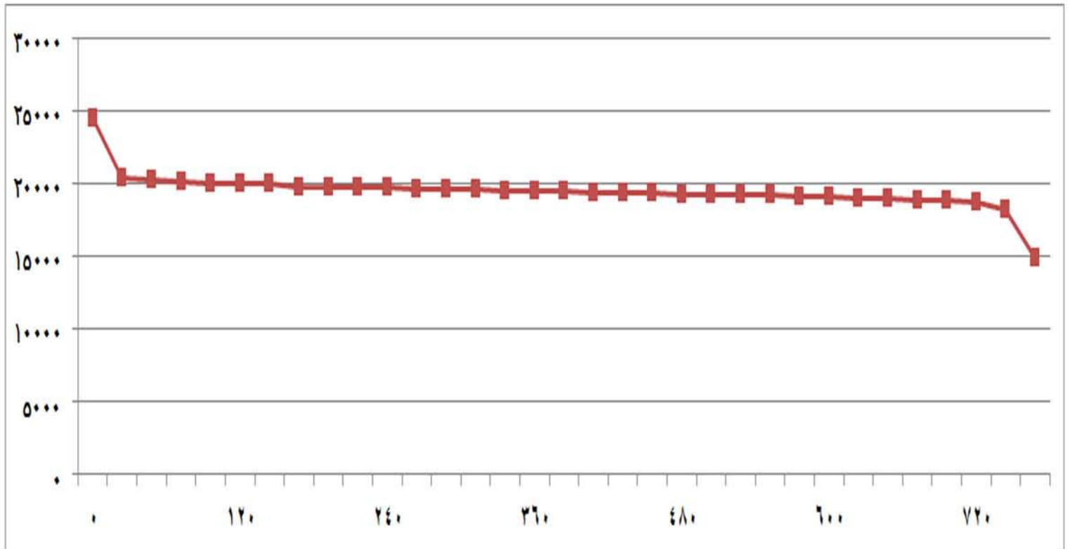
شكل (٨) المنحنى الشهري لفترة الحمل ديسمبر ٢٠١٦
