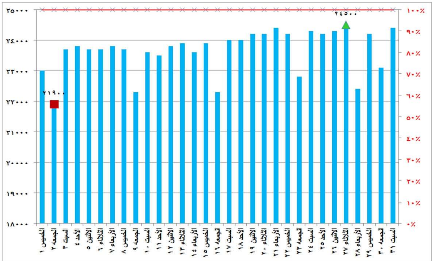
شكل (٥) قدرات الانتاج المتاحة ونسبتها للحمل الأقصى خلال شهر ديسمبر ٢٠١٦
