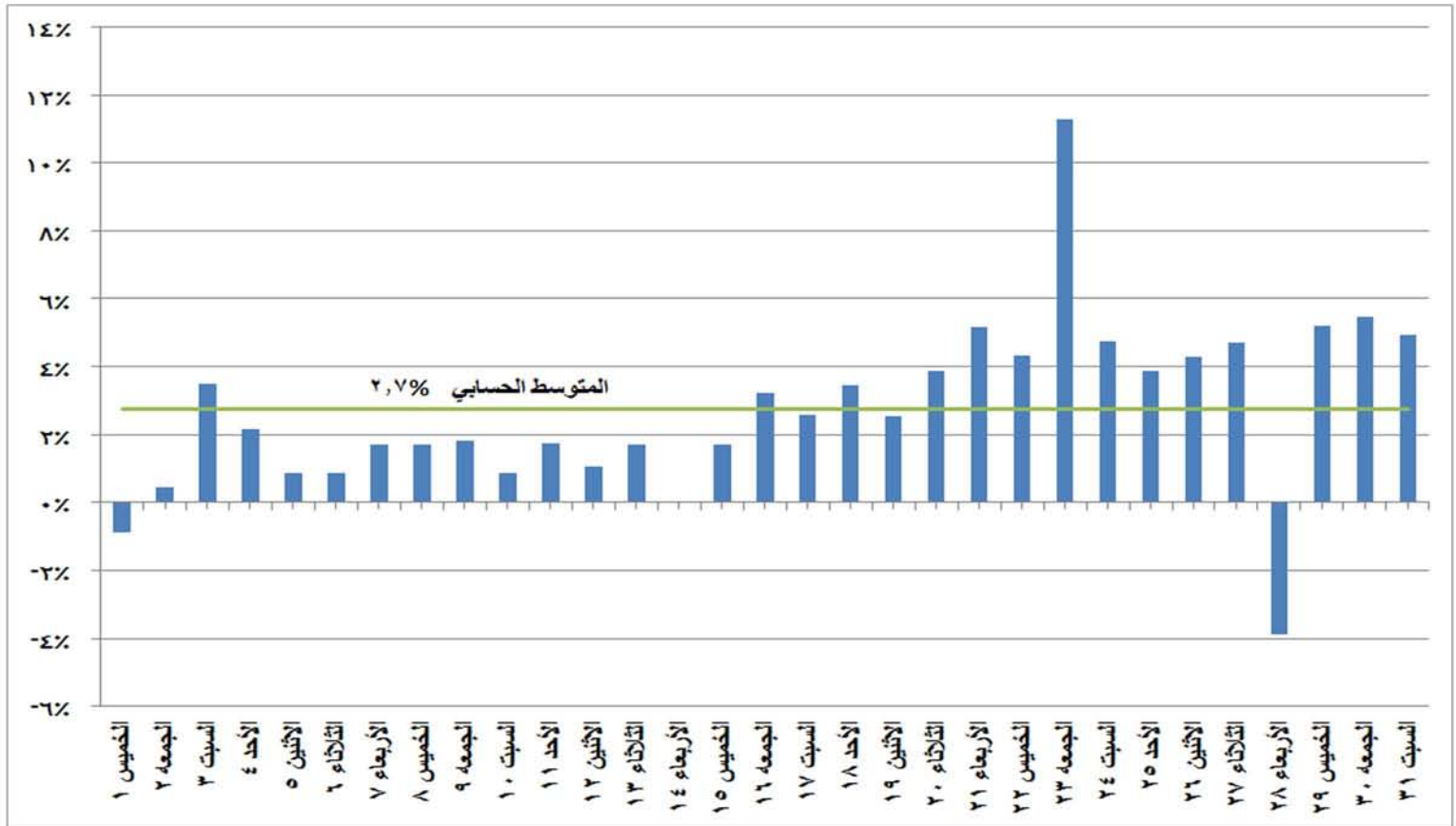
شكل (٩) النسب المئوية للتغير في الحمل الاقصى خلال شهر ديسمبر ٢٠١٦ مقارنة باليوم المماثل من العام الماضي
