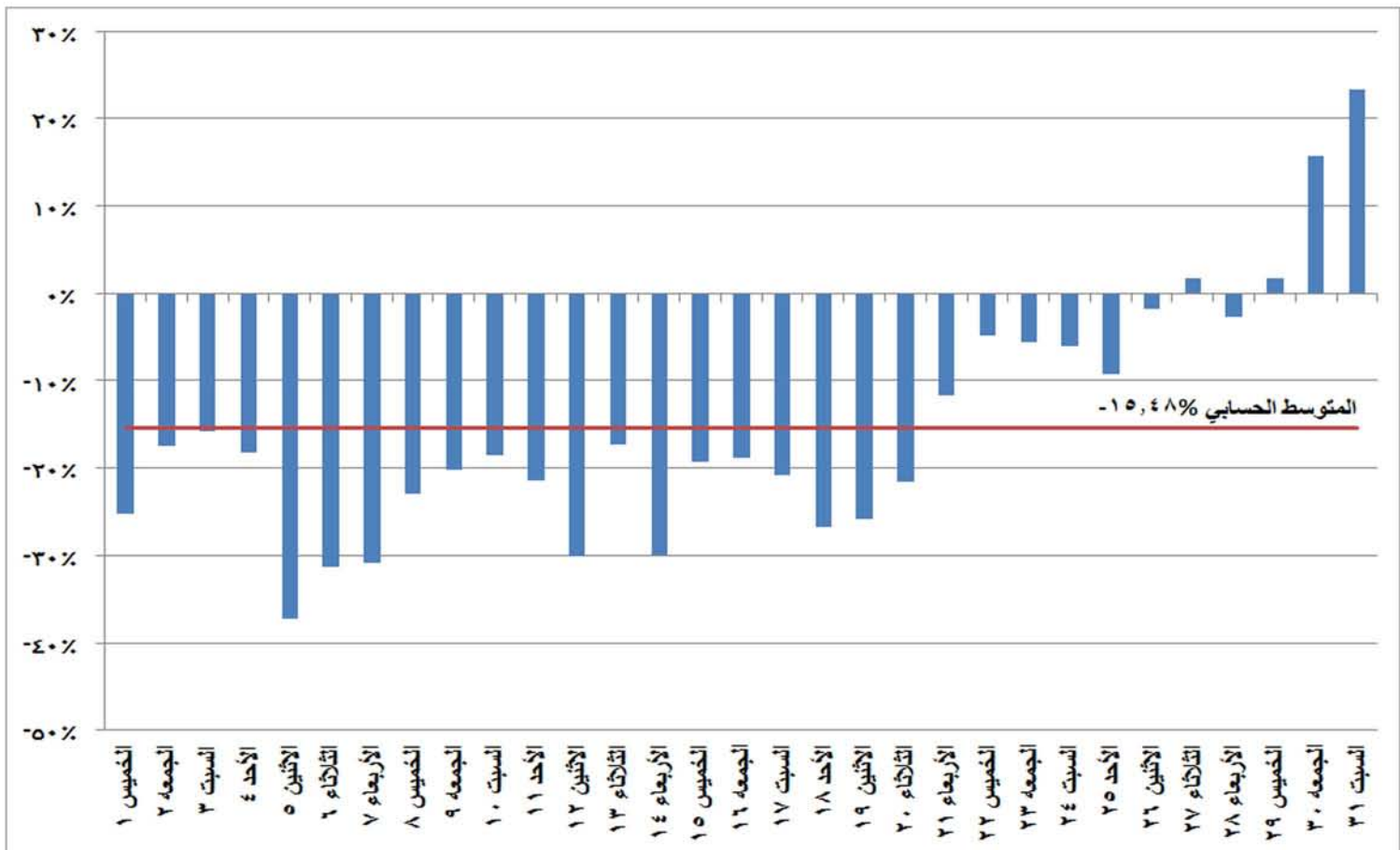
شكل (٢٠) نسب التغير في استخدام المازوت في إنتاج الطاقة الكهربائية خلال شهر ديسمبر ٢٠١٦ مقارنة بالشهر المماثل من العام السابق
