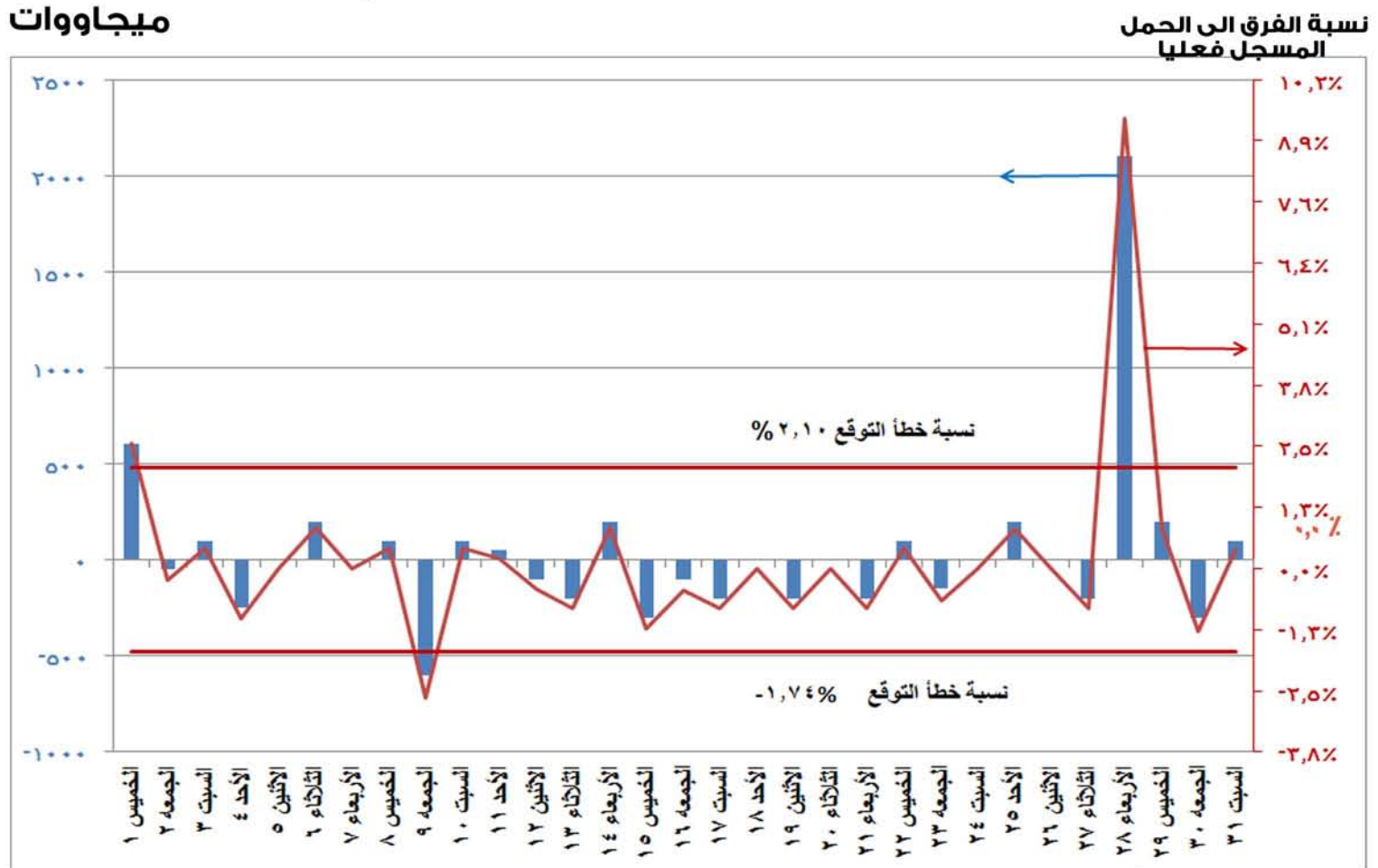
شكل (١٠) الفرق بين الحمل الأقصى المتوقع والمسجل فعلياً ونسبة الفرق إلى الحمل المسجل فعلياً خلال شهر ديسمبر ٢٠١٦
