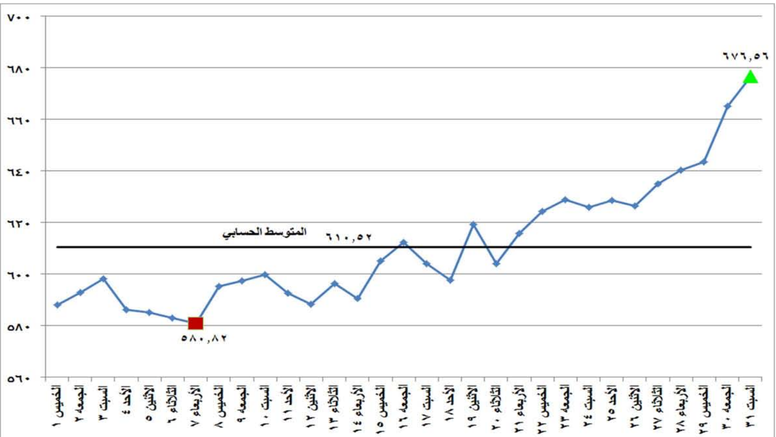
شكل (١٤) معامل انبعاثات غاز ثاني اكسيد الكربون المكافئ على مدى شهر ديسمبر ٢٠١٦
