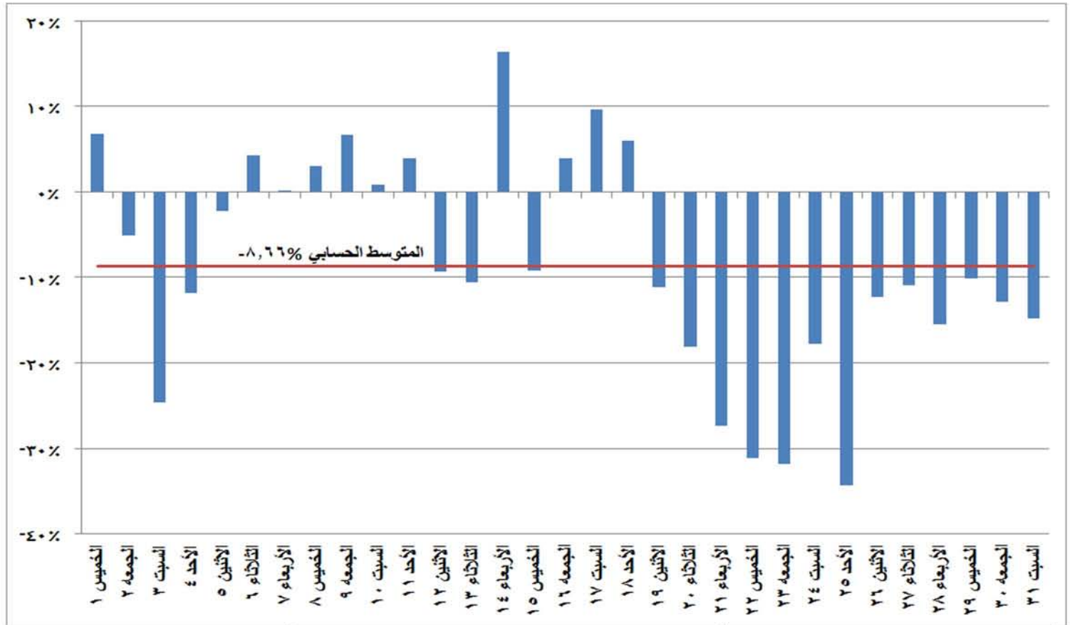
شكل (٢٢) نسب التغير في استخدام المصادر غير الحرارية في إنتاج الطاقة الكهربائية خلال شهر ديسمبر ٢٠١٦ مقارنة بالشهر المماثل من العام السابق
