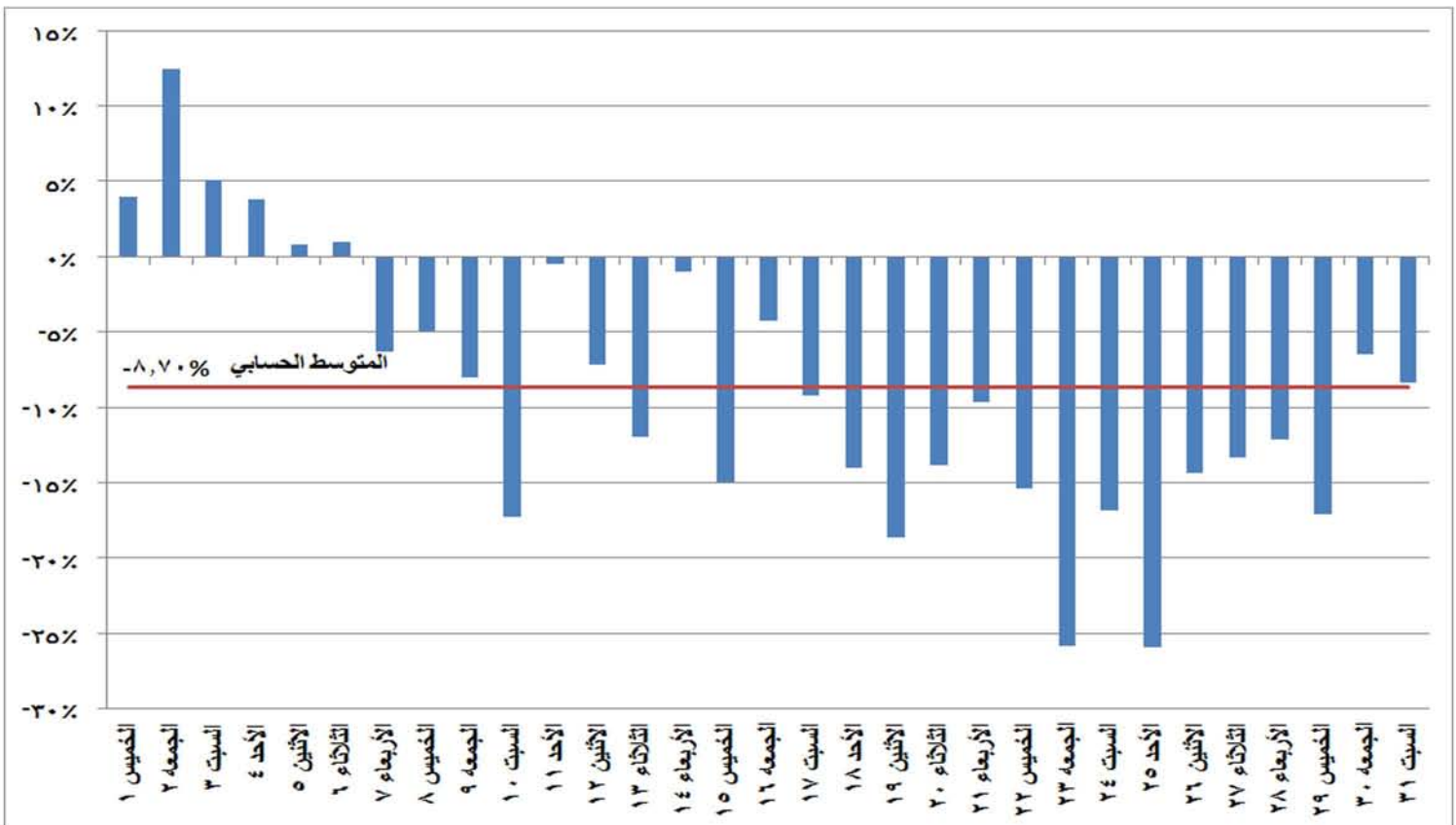
شكل (٢٤) نسب التغير في استخدام المصادر المائية في إنتاج الطاقة الكهربائية خلال شهر ديسمبر ٢٠١٦ مقارنة بالشهر المماثل من العام السابق
