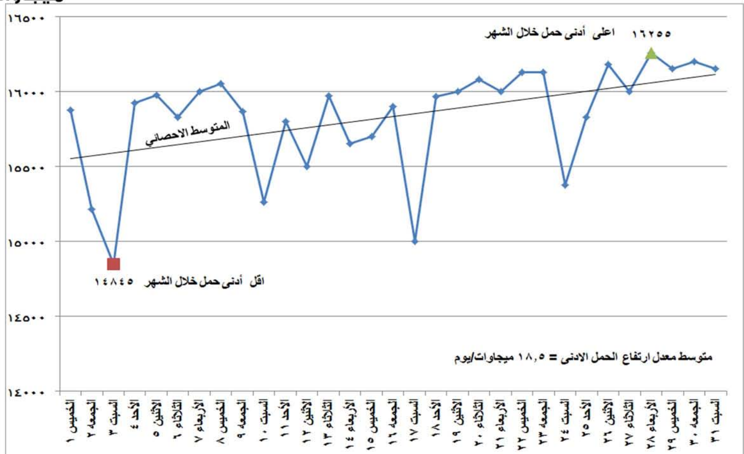
شكل (٢) تطور الحمل الادنى اليومي خلال شهر ديسمبر ٢٠١٦
