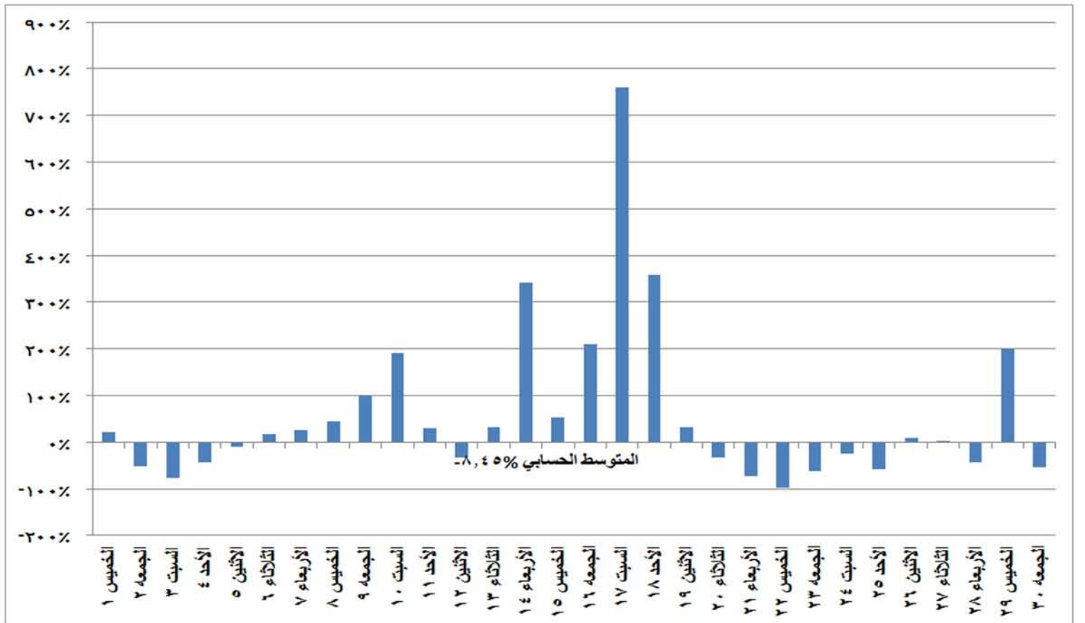
شكل (٢٦) نسب التغير في استخدام الرياح والشمس في إنتاج الطاقة الكهربائية خلال شهر ديسمبر ٢٠١٦ مقارنة بالشهر المماثل من العام السابق
