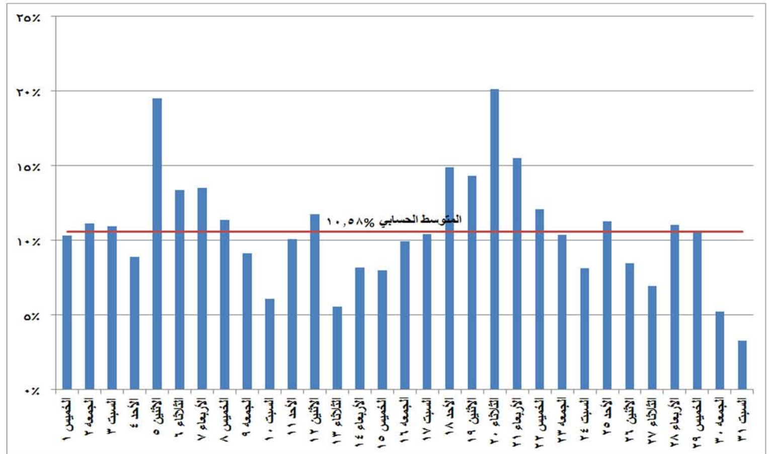
شكل (١٨) نسب التغير في استخدام الغاز الطبيعي في إنتاج الطاقة الكهربائية خلال شهر ديسمبر ٢٠١٦ مقارنة بالشهر المماثل من العام السابق
