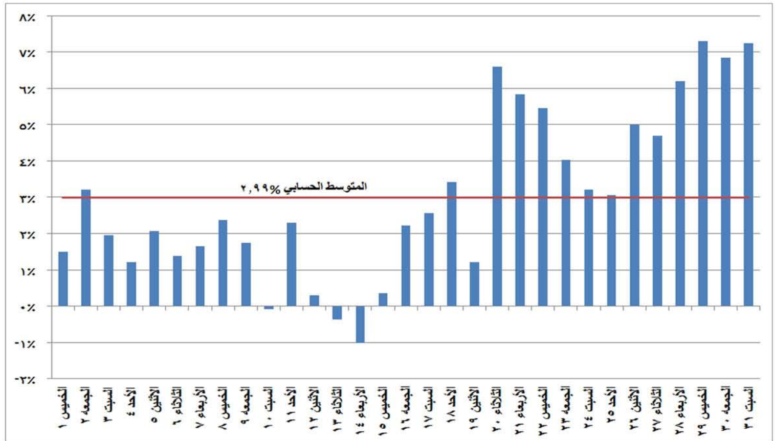
شكل (١٦) نسب التغير في الطاقة الكهربائية المنتجة خلال شهر ديسمبر ٢٠١٦ مقارنة بالشهر المماثل من العام السابق
