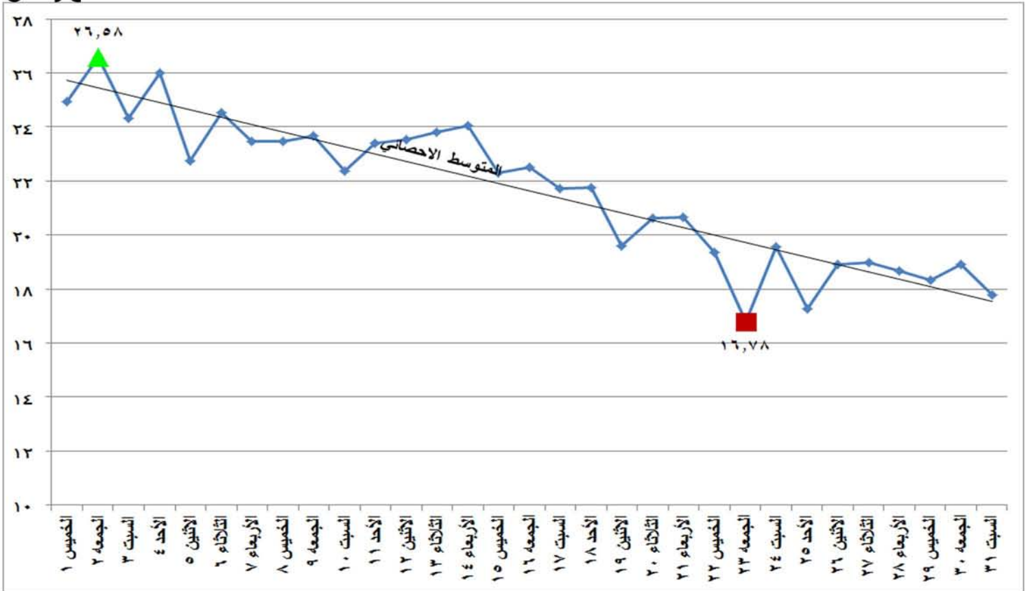
شكل (٢٣) الطاقة الكهربائية المنتجة من المصادر المائية خلال شهر ديسمبر ٢٠١٦
